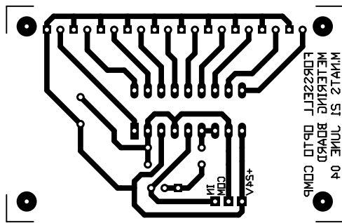
FORSSE~2 Bottom Layer
